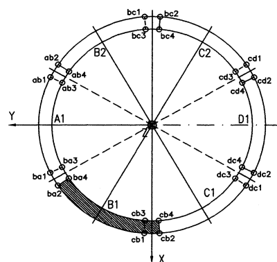
vue frontale de l'anneau de voussoir
