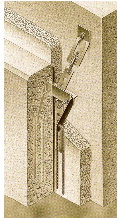
Systèmes d'ancrages de façades
