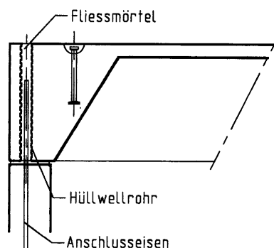
Anschlussdetail Rippenplatte-Wand mit Endblockausbildung
