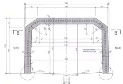
Querschnitt
